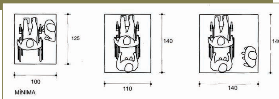
Dimensiones mínimas recomendadas para la cabina del ascensor.
